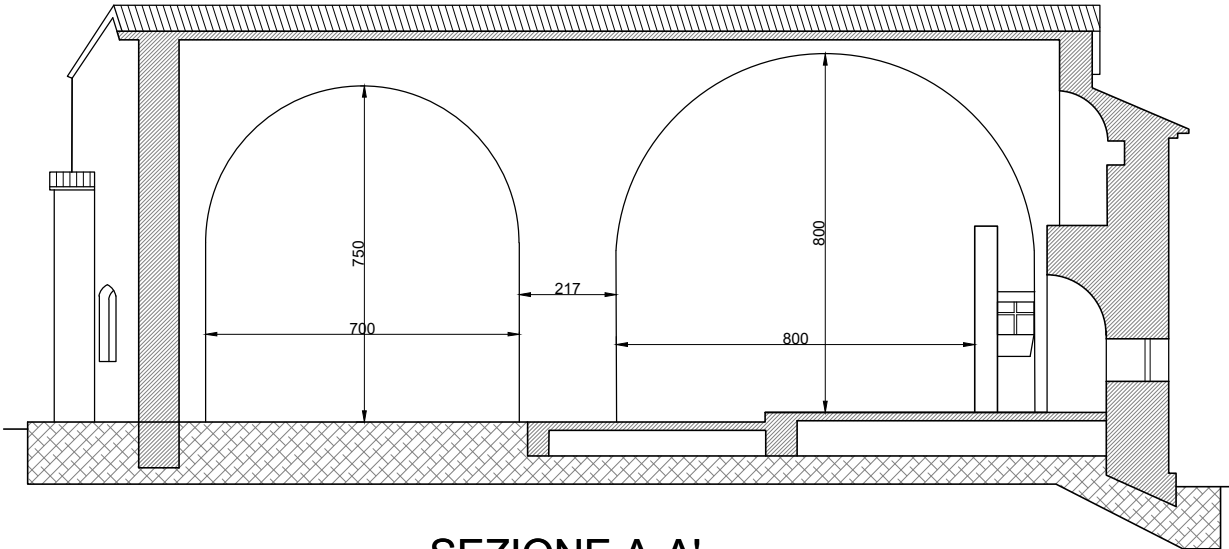
SEZIONE A-A'
